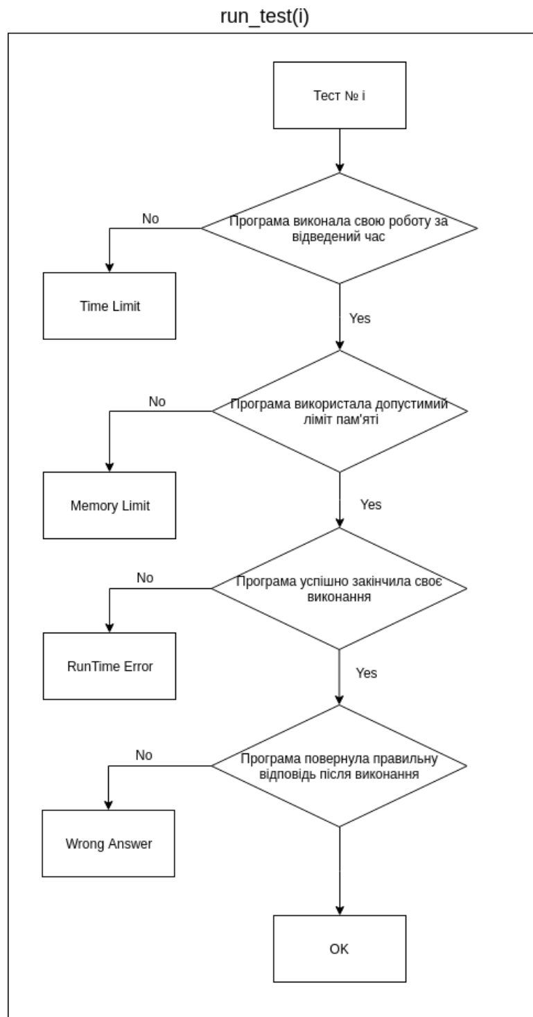
Рисунок 3 - Схема тестування на заданому тесті
