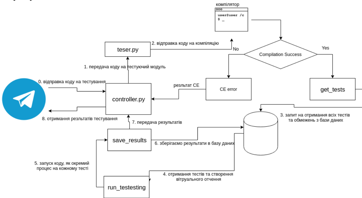
Рисунок 1 - Логіка роботи тестувального модуля
