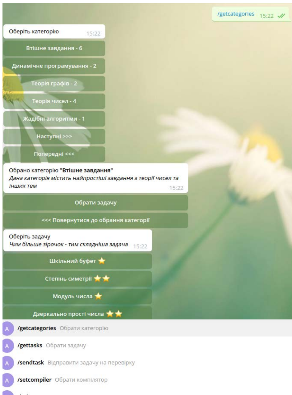
Рисунок 4 - Діалог з ботом, та можливі команди
