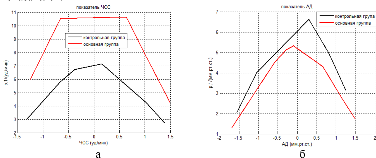
Рис. 4. Применение стандартизированной оценки распределения показателей ЧСС (а) и АД (б) контрольной и основной групп
