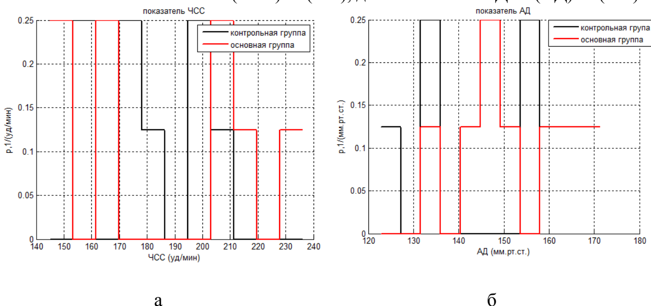
Рис. 1. Гистограммы распределения показателя ЧСС (а) и АД (б) контрольной и основной группы для определения информативности по модифицированному критерию Колмогорова-Смирнова
