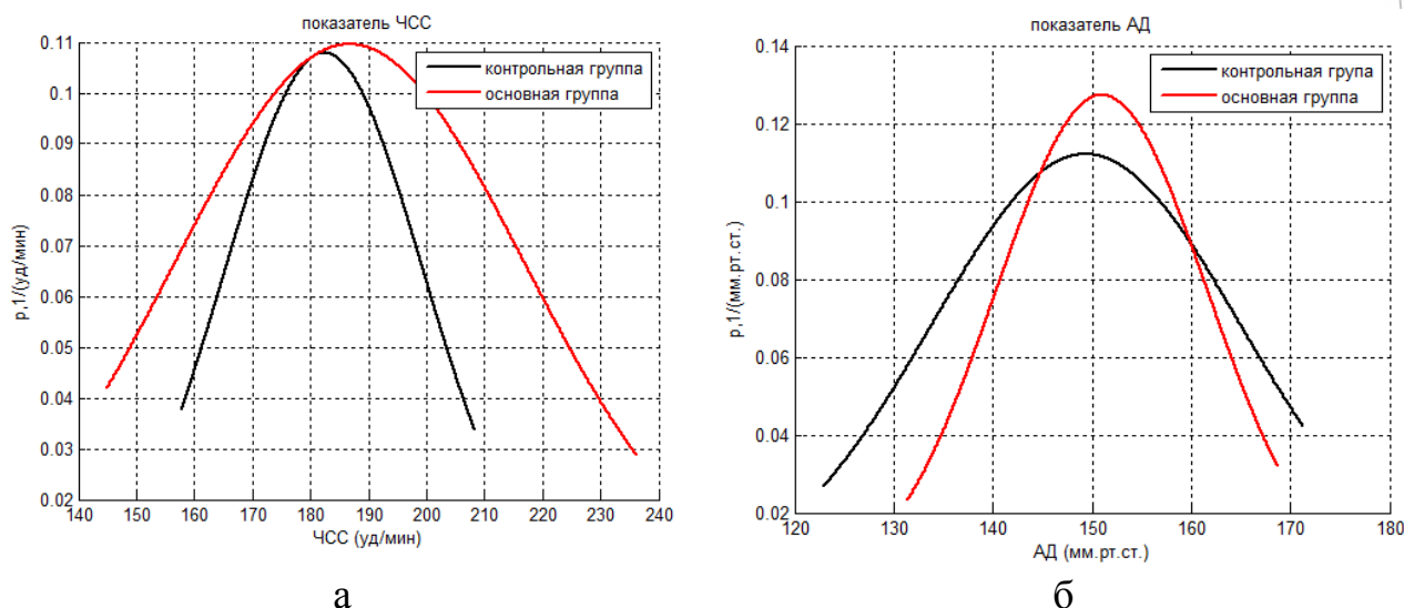
Рис. 3. Теоретические нормальные законы распределения показателей ЧСС (а) и АД (б) контрольной и основной групп
