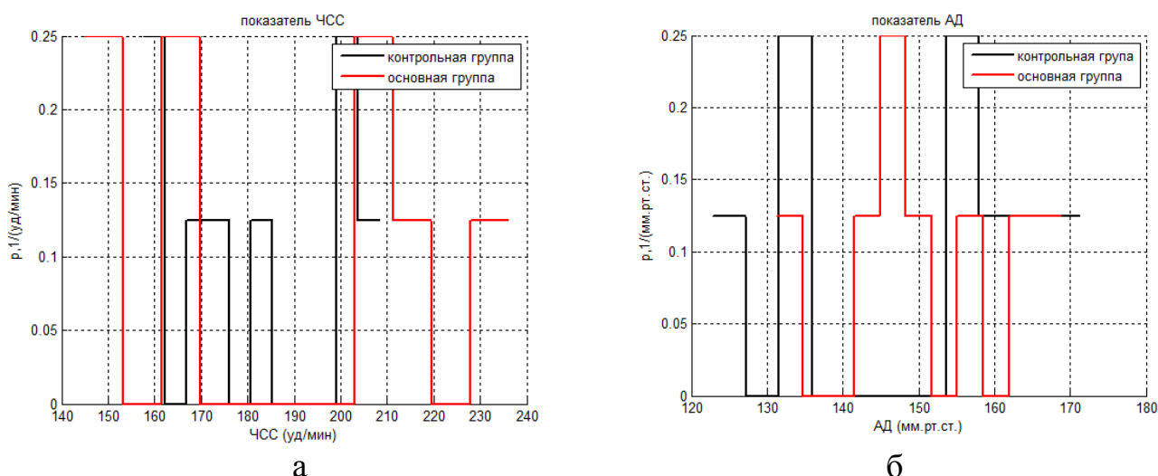
Рис. 2. Гистограммы распределения показателя ЧСС (а) и АД (б) контрольной и основной группы для определения информативности по энтропийной мере Шеннона
