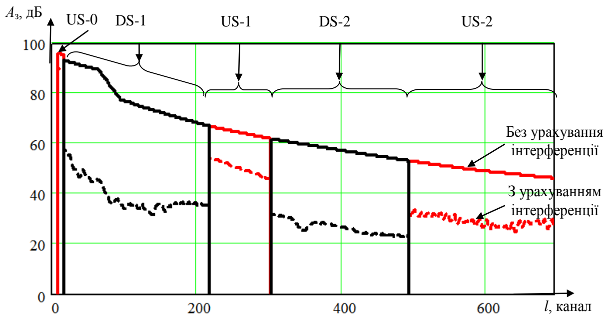
Рис. 2. Порівняння розподілу по каналах СП VDSL2 захищеності сигналу від завад з урахуванням інтерференції та за її відсутності ( l_{л}=500 м)
