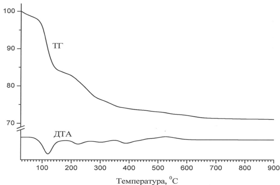
Рис. 1. Кривые ТГ и ДТА для бруситфосфатной связки
