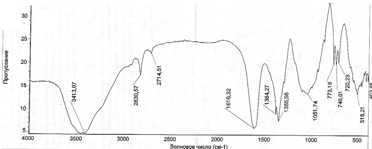
Рис. 2. ИК-спектр для бруситфосфатной связки, обожженной при 900 °С Авторская разработка
