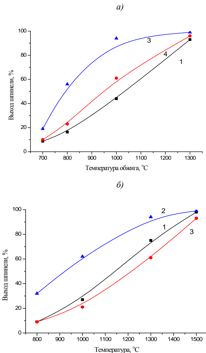
Рис. 2. Влияние температуры и способа подготовки смесей Mg(OH)_2 + Cr(OH)_3 (а), MgO + Cr_2O_3 (б), MgO + Al_2O_3 (в) на выход шпинели: 1 - простое смешение компонентов; 2 – предварительная совместная обработка компонентов в ПМ; 3 – совместное истирание компонентов в ШКМ; 4 – истирание MgO в ШКМ перед смешением компонентов Авторская разработка
