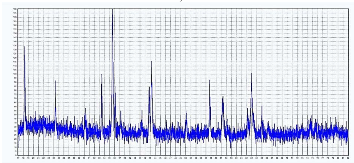
Рис. 1. Дифрактограммы продукта обжига (800 °С, 1 ч) смесей Mg(OH)_2 и Cr(OH)_3 , полученных без механической обработки (а), обработкой в ШКМ (б) и ПМ (в)
