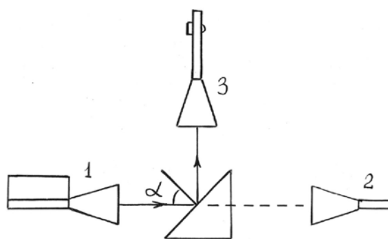
Рис.2 Схема установки для наблюдения аналога туннельного эффекта
