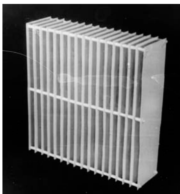
Рис.5 Металлоленточная структура
