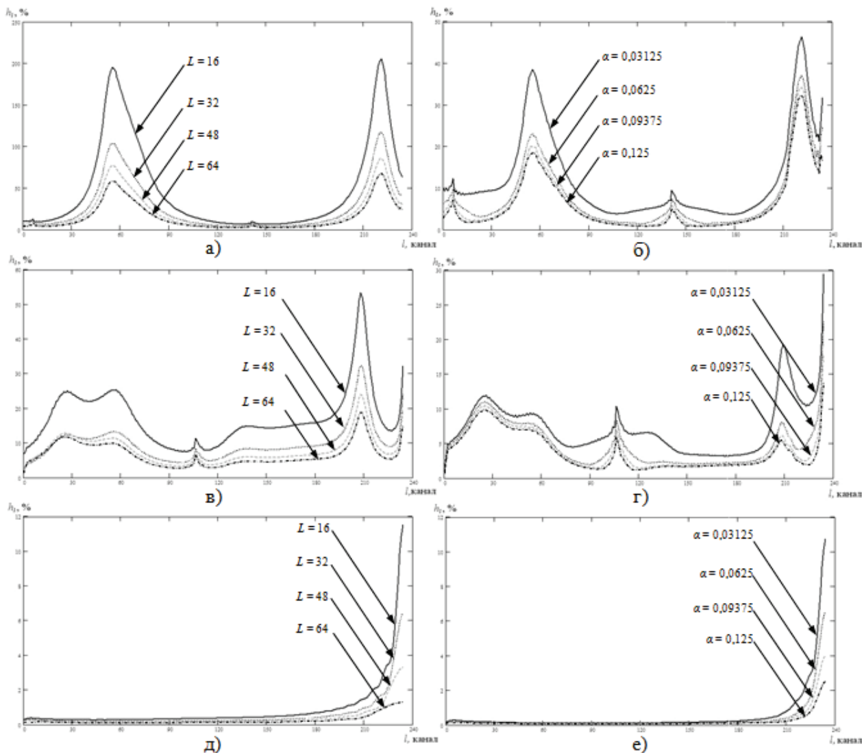
Рисунок 3 – Графічне зображення залежності h від l (навантаження являє собою ємність ( C = 1 нФ):
