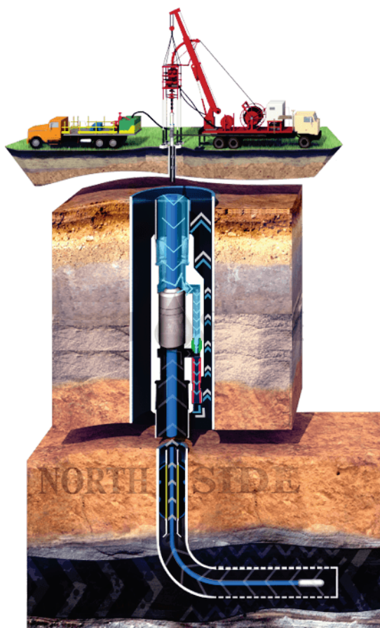
Рис.1. Схема розміщення обладнання колтубінг при дослідженні та експлуатації горизонтальної свердловини зі струминним насосом.
